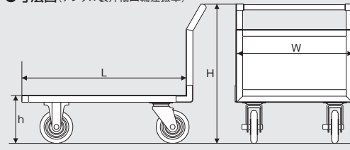
●寸法図(アングル製片袖四輪運搬車)
